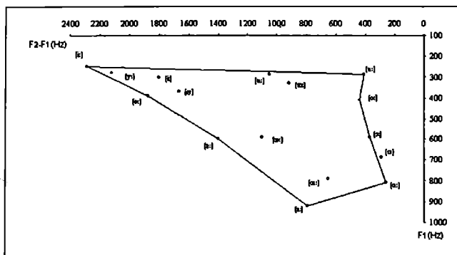
4 p a v. Kardinalinių pirminių (•) ir antrinių (○) balsių spektro charakteristikos (II variantas)
