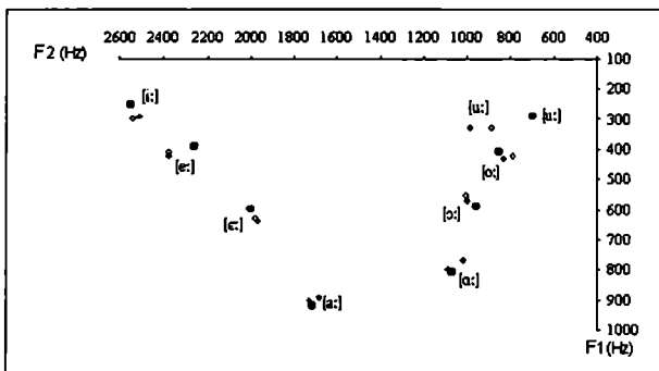
5 pav. Pirminiai kardinaliniai balsiai, ištarti neutralia (●), kylančia (♦) ir krinantčia (○) intonacija
