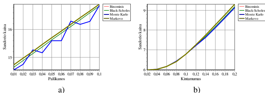
2 pav. Sandorio kainos priklausomybė nuo jo parametru.
