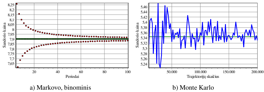
3 pav. Modelių konvergavimas.
