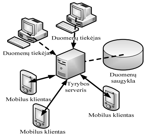
1 pav. Mobiliosios tyrybos sistemos architektūra (Domenico, Paolo, 2010)
